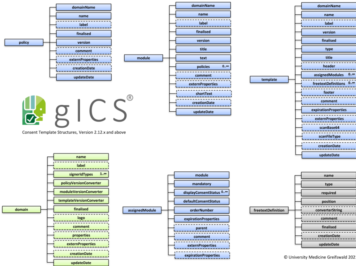
Abbildung 7-1: Überblick der Attribute, welche bei den jeweiligen Bausteinen gesetzt werden können. Attribute mit gestrichelten Rand sind optional, alle anderen sind Pflichtattribute und müssen (zumindest leer) gesetzt werden.
