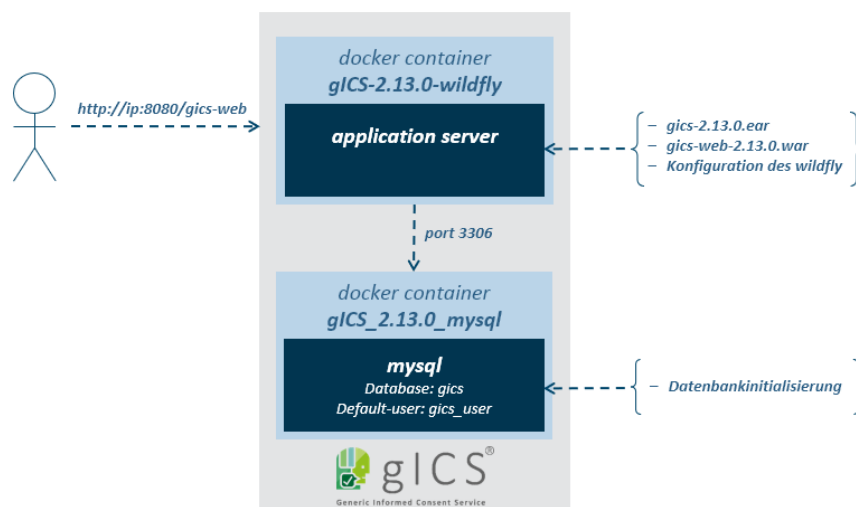
Abbildung 6-1: Aktuelle Architektur des gICS Docker Containers am Beispiel der Version 2.13.0.
